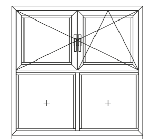
Ein Drehflügel, ein Dreh-Kippflügel und zwei feste Flügel
