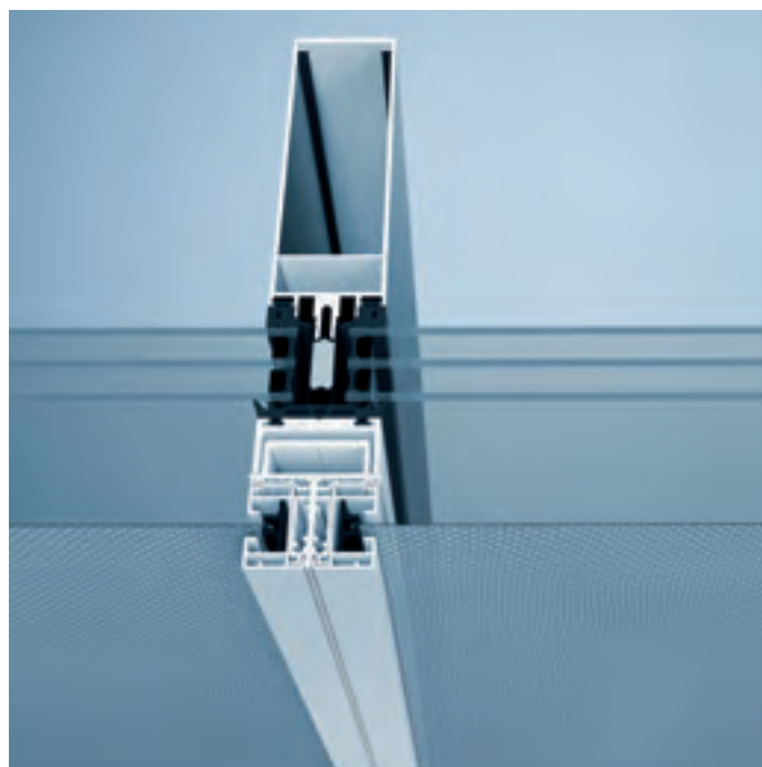
Částečně integrovaný fasádní systém protisluneční ochrany heroal VS Z CS
