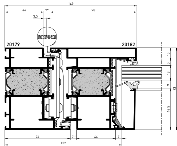
Innenanwendung
