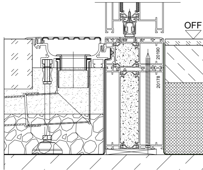
Außenanwendung
